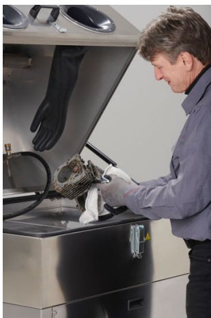
De poetsdoek en hogedrukreiniger kunnen samen worden gebruikt om een sterk vervuild motoronderdeel te reinigen. (Foto: Mewa)
